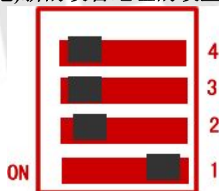
S2 地址为1拨码设置
