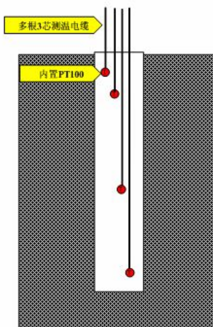
布线方式
