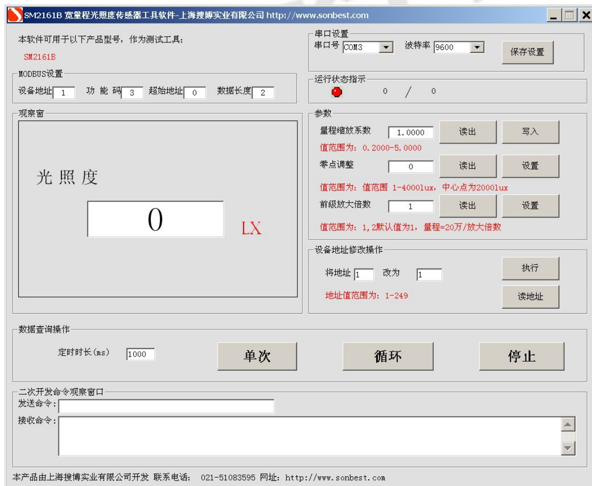
图 3.1 软件界面
