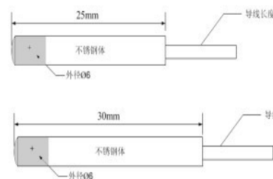
传感器外形尺寸
