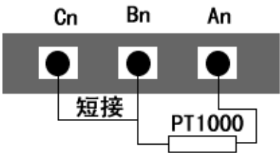
二线制接法
