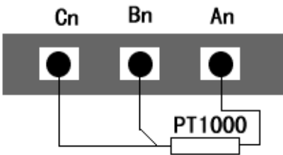
三线制接法
