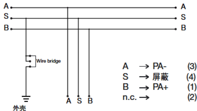
1 支线输出接线图
