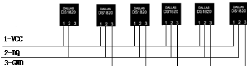
SLIT1-1 总线接线图
